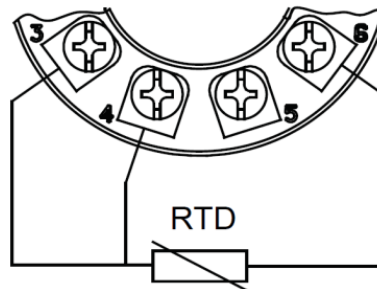
3-Leiter-Kompensation
